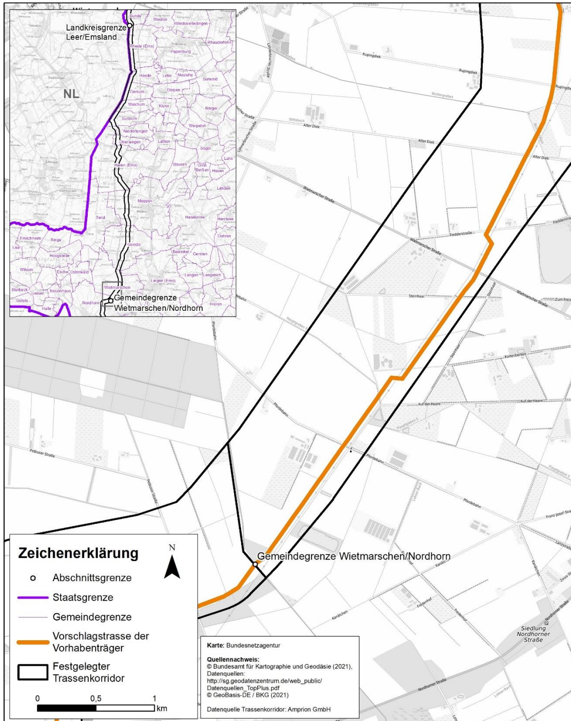
Abb. 2: Aktualisierter Trassenverlauf auf dem Gemeindegebiet von Wietmarschen
