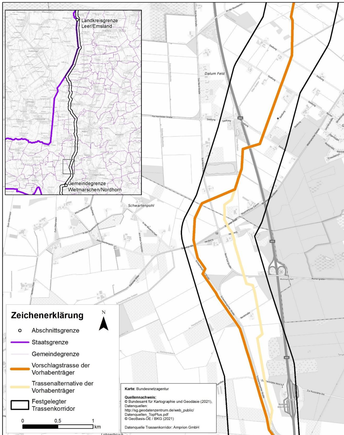
Abb. 1: Aktualisierter Trassenverlauf auf den Gemeindegebieten von Geeste/Wietmarschen
