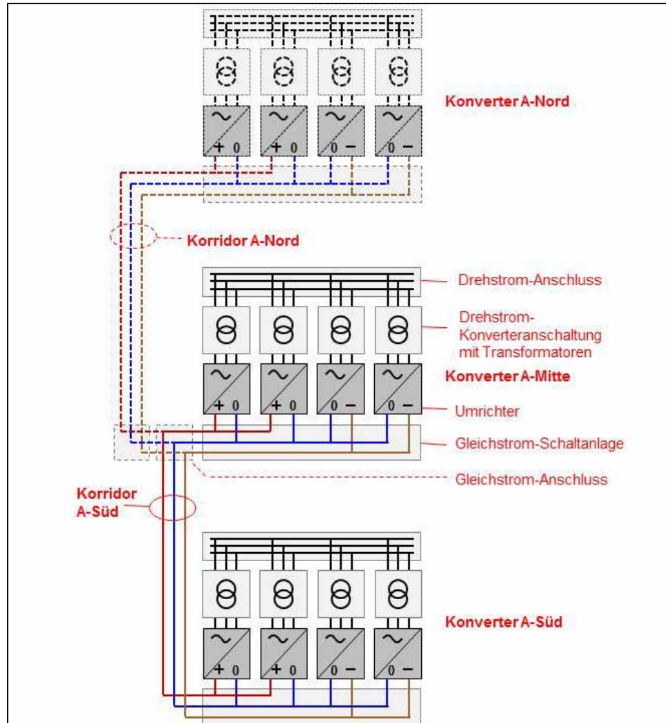
Abbildung 2-10 Schematische Darstellung der Funktionsblöcke der Konverterstation und des Gesamtkorridors A
