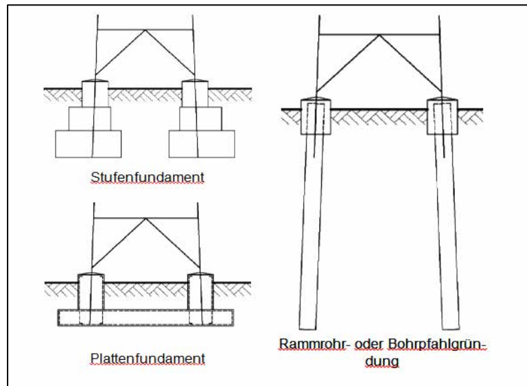
Abbildung 2-6 Prinzipzeichnung unterschiedlicher Mastformen (Tragmast)
