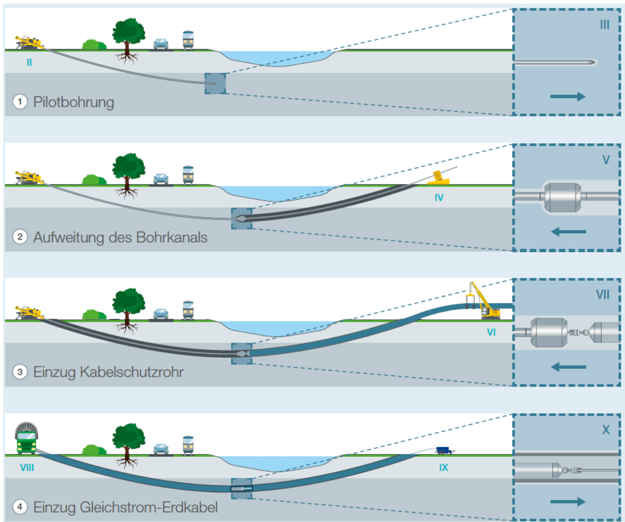
Abbildung 17: Beispiel HDD-Verfahren
