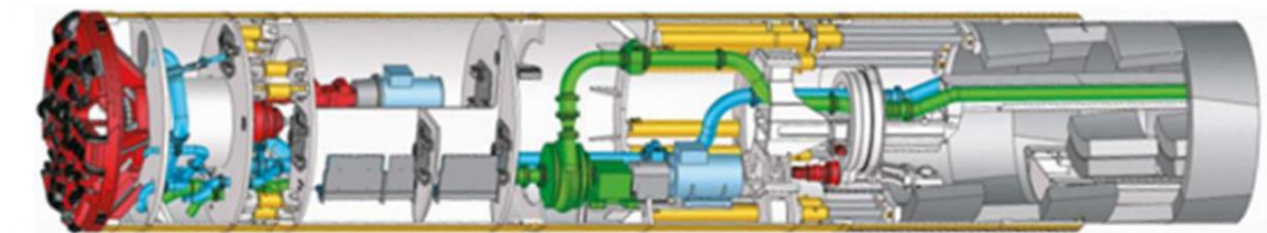
Abbildung 25: Tübbingvortriebsmaschine
