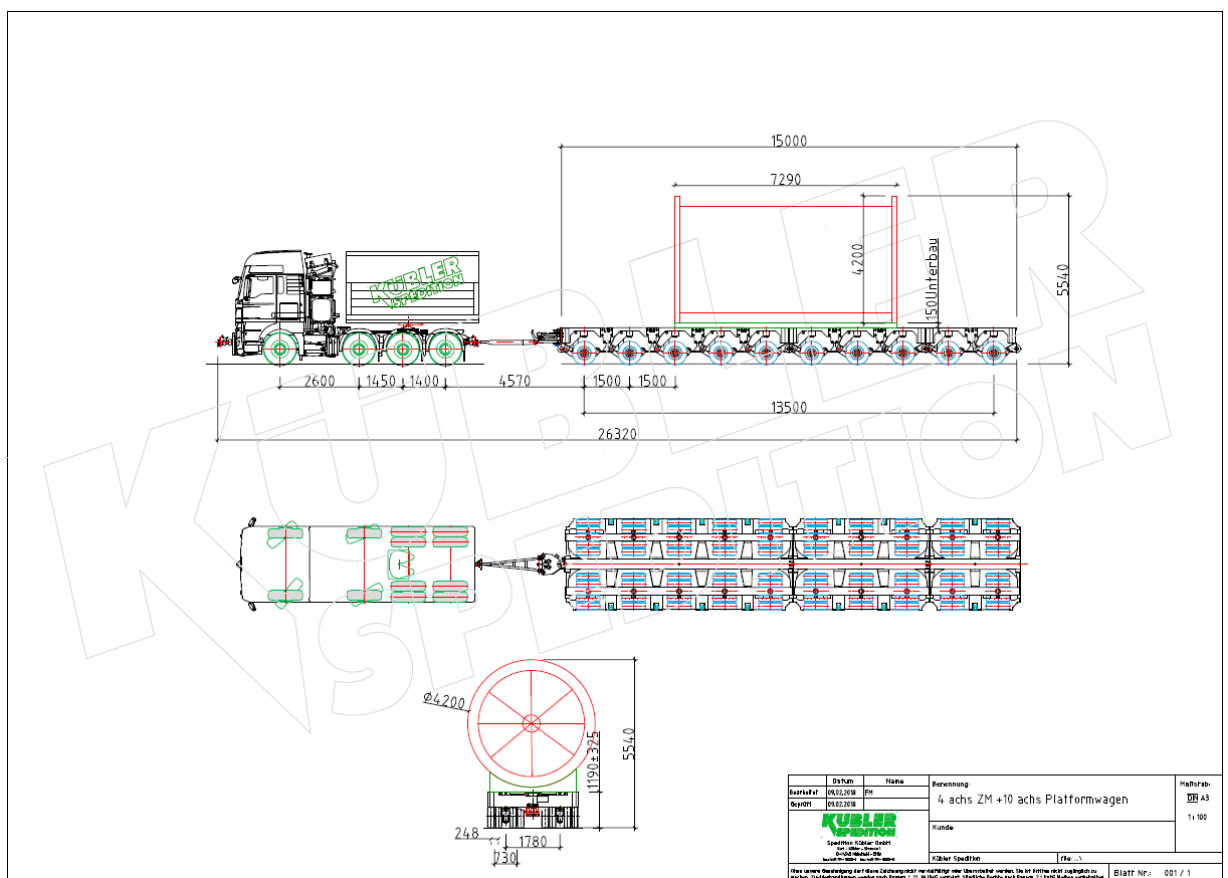
Abbildung 10: Skizze Plateau-Fahrzeug
