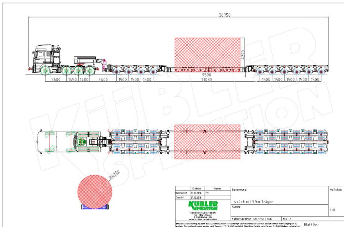
Abbildung 6: Skizze Kesselbrücke
