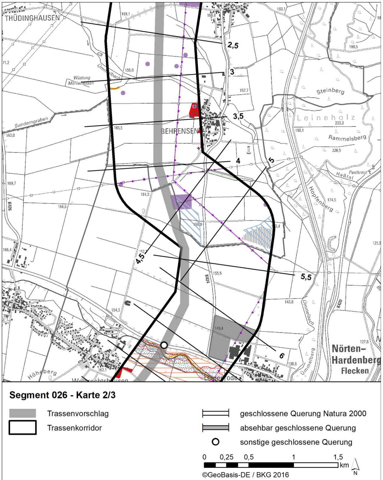
Abbildung 24: Segment 026 km 2,5 bis km 6,5 – Karte 2/3
