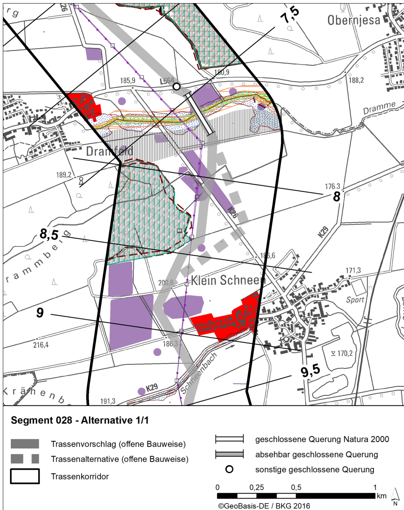
Abbildung 32: Trassenverlauf des Trassenvorschlags und der Alternative 1/1
