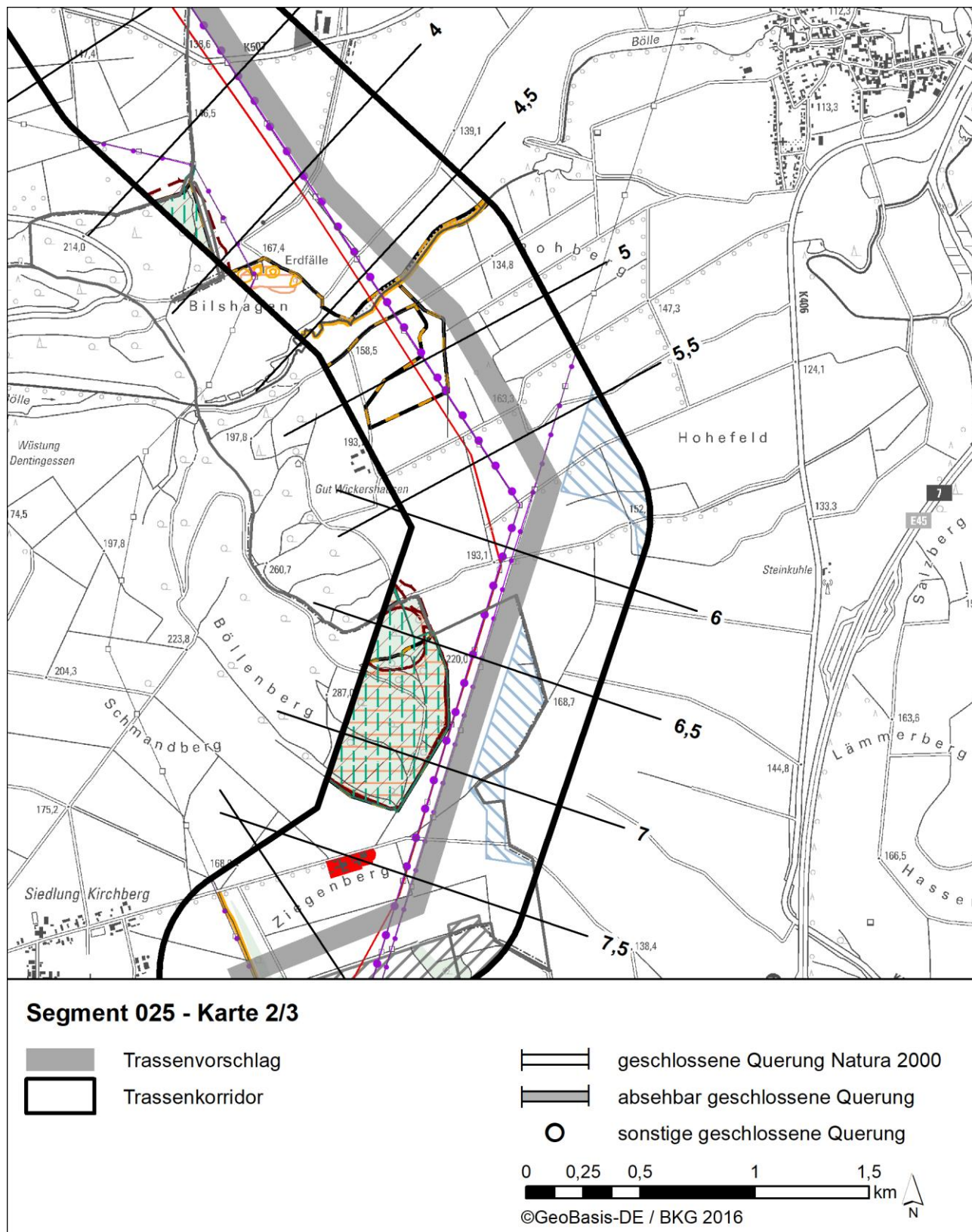
Abbildung 21: Segment 025 km 4,0 bis km 7,5 – Karte 2/3
