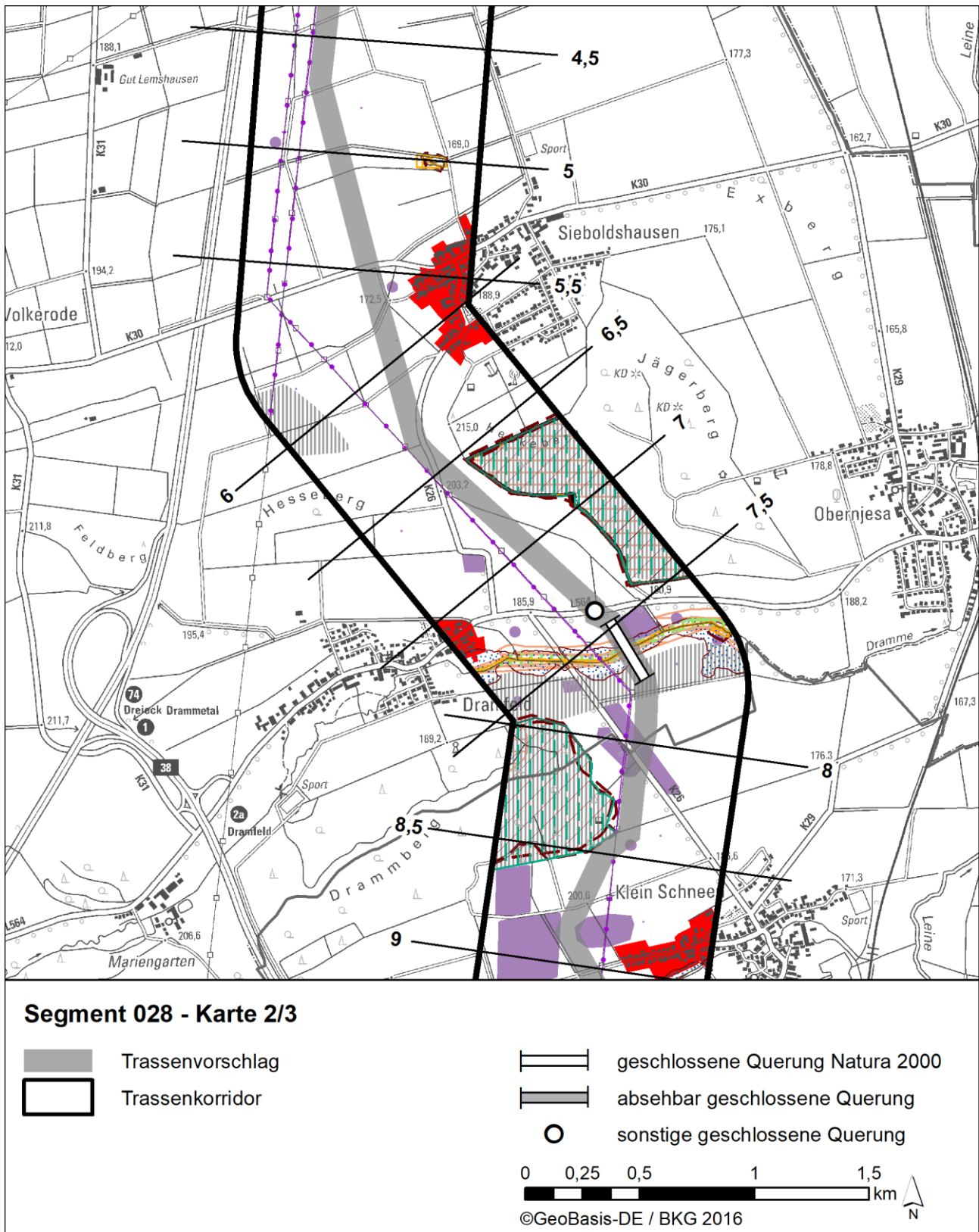
Abbildung 30: Segment 028 km 4,5 bis km 9,0 – Karte 2/3
