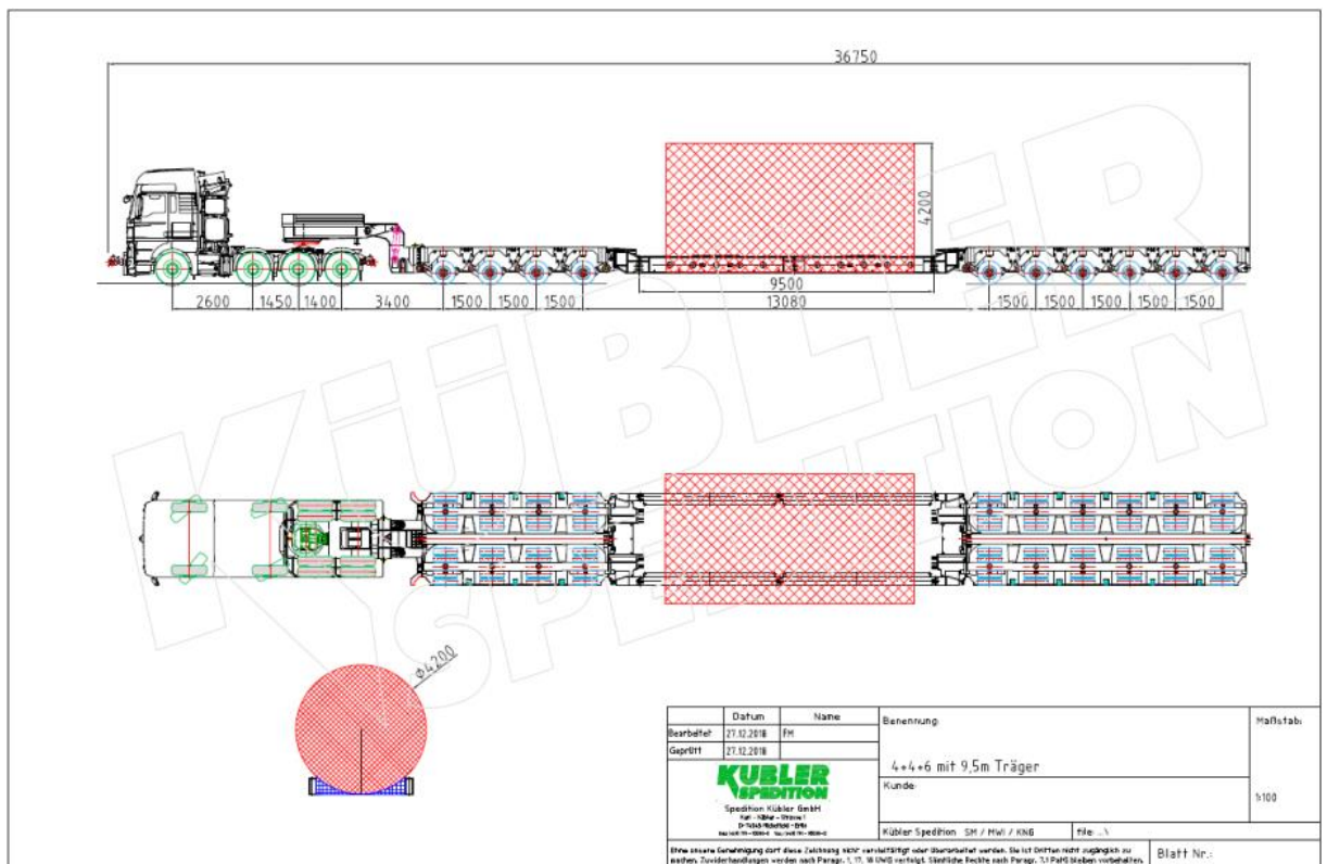
Abbildung 6: Skizze Kesselbrücke
