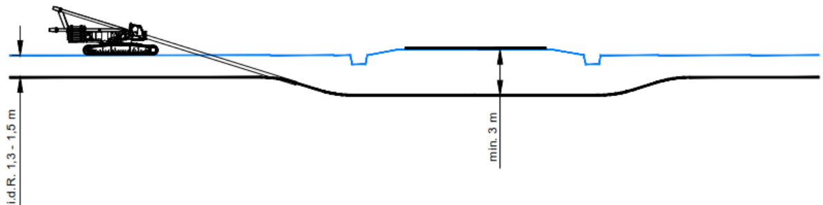
Abbildung 18: Typische Mindestüberdeckungen bei HDD-Querungen
