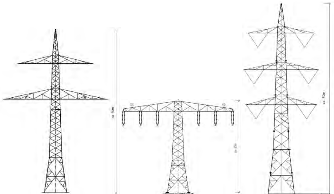
Abbildung 33: Schematische Darstellung dreier herkömmlicher Stahlgittermastformen
