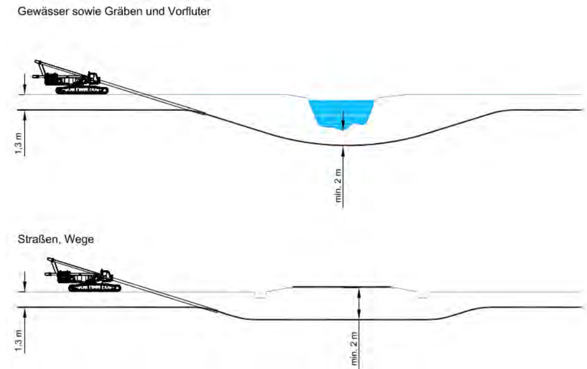
Abbildung 21: Typische Mindestüberdeckungen bei HDD-Querungen
