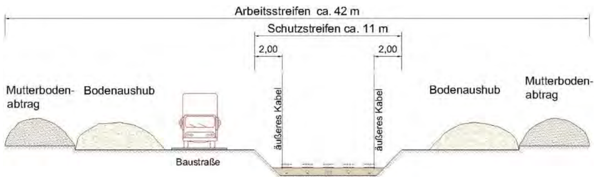
Abbildung 13: Musterquerschnitt für 525 kV, zwei Kabel/Schutzrohre in einem Graben
