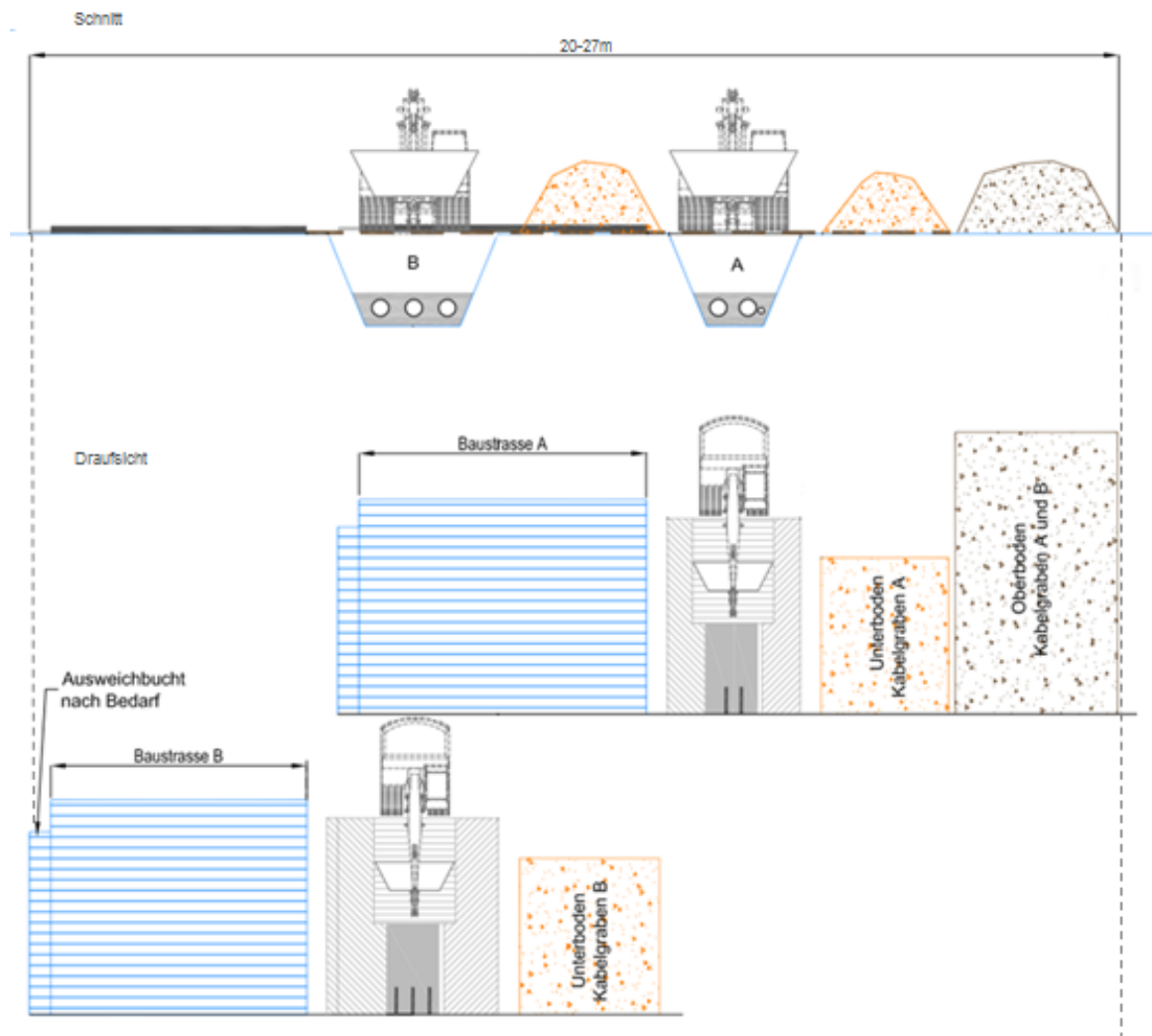
Abbildung 17: Mögliche verringerte Arbeitsstreifenbreiten in Bereichen von Engstellen; hier: Öffnen und Schließen der Kabelgräben A und B in versetzter Bauweise sowie Versetzen der Baustraße
