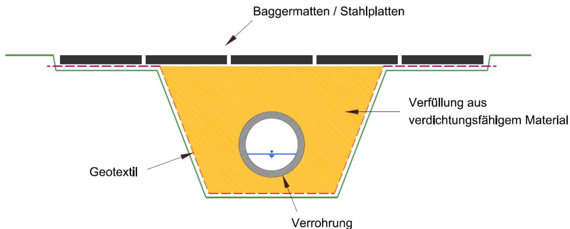
Abb. 9: Prinzipskizze Grabenverrohrung
