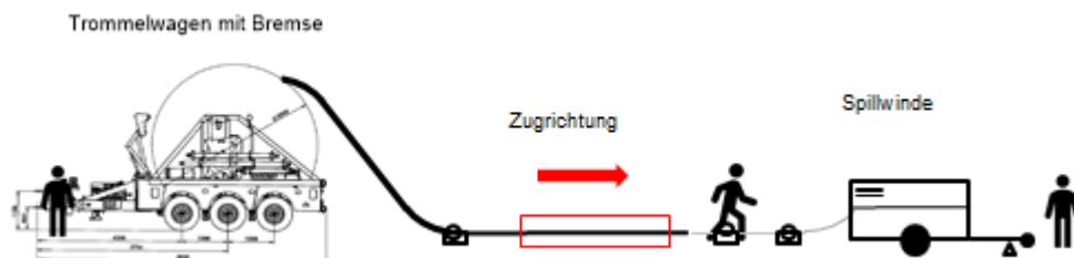
Abb. 19: Geschlossene Kabelverlegung (Rohranlage)
