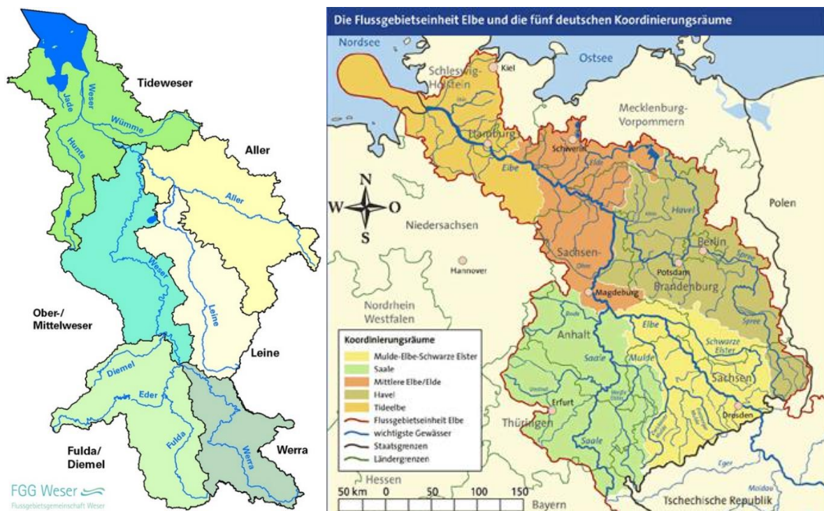
Abb. 1: Flussgebietseinheiten Weser und Elbe mit Koordinierungsräumen ( https://www.fgg-weser.de/ / https://www.fgg-elbe.de/fgg_elbe.html , Datum des Zugriffs 24.08.2021)
