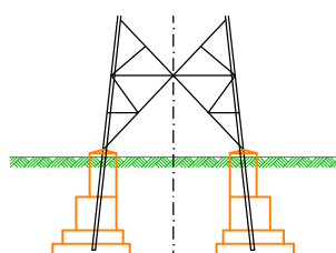
Stufenfundament
