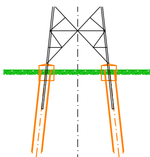
Rammfundament
