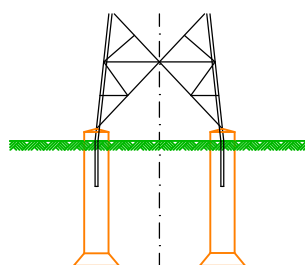
Bohrfundament
