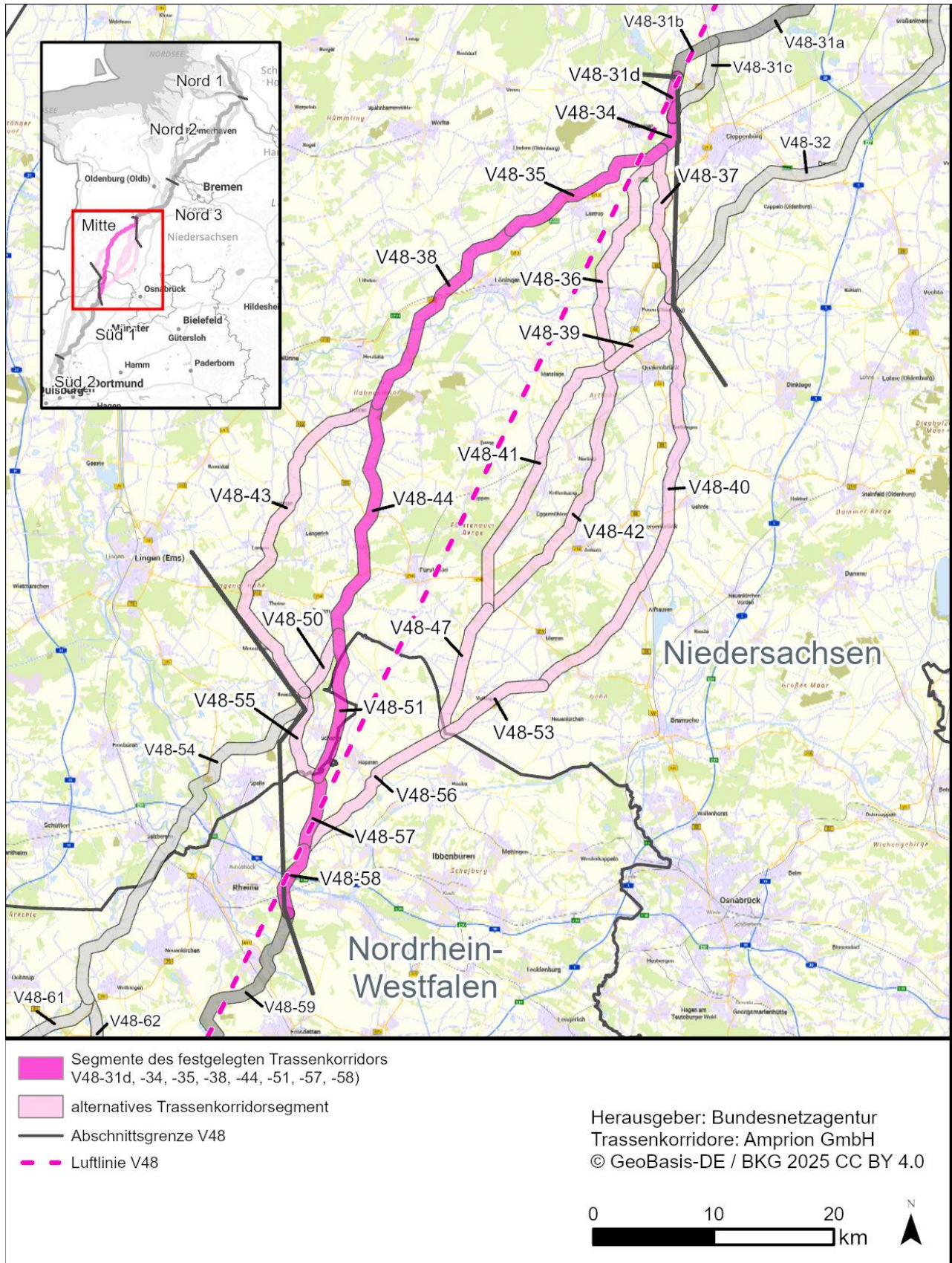
Abbildung 1: Festgelegter Trassenkorridor
