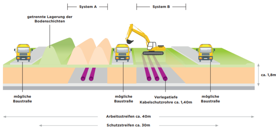
Abb. 2-3: Schematische Darstellung des Arbeitstreifens für das Einzelsystem (Einzelvorhaben (Quelle: Amprion GmbH)
